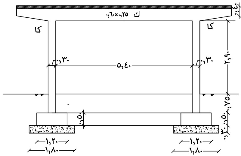
قطاع راسي
