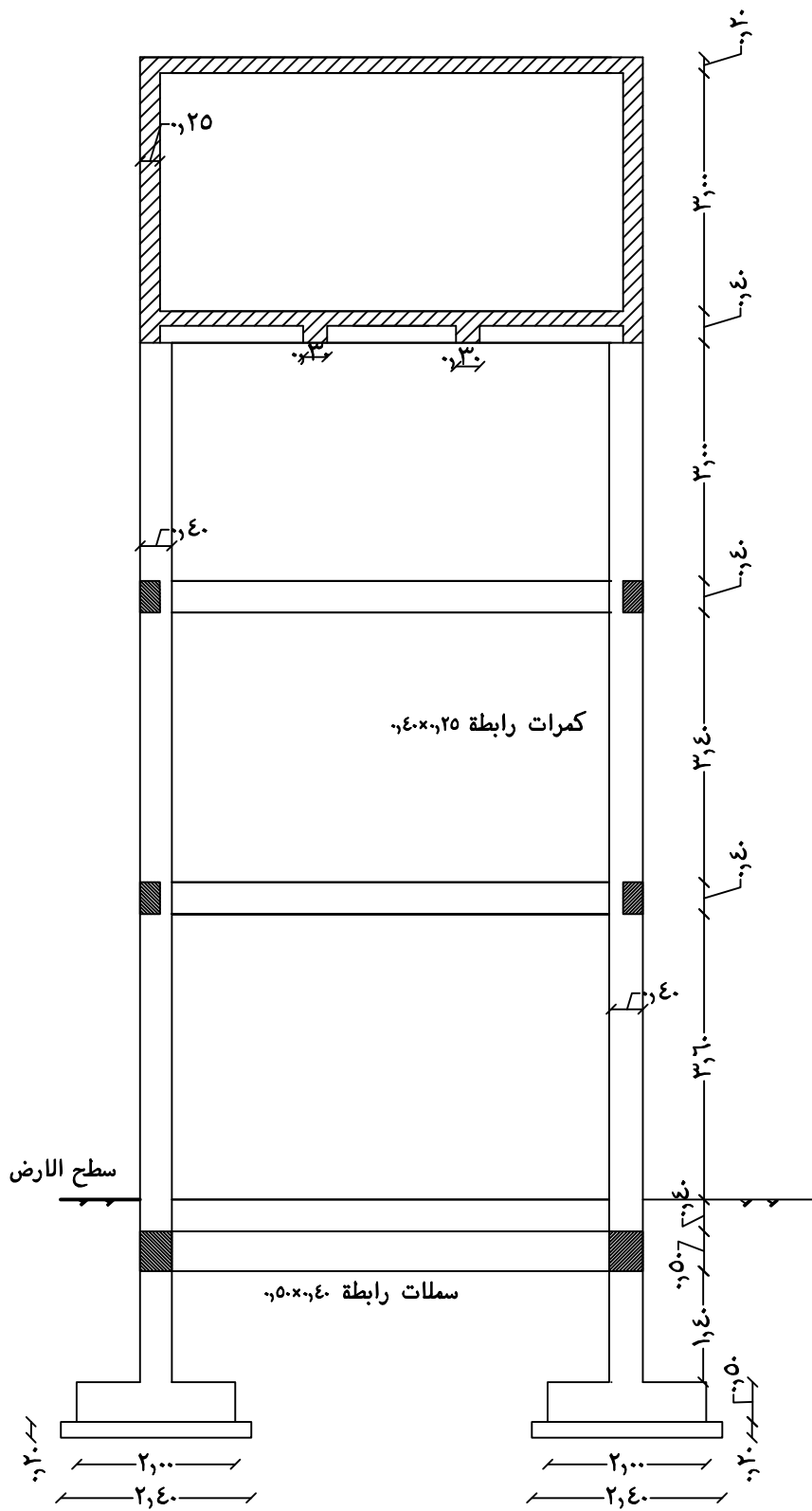
قطاع راسي
