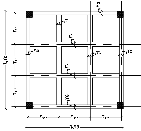
مسقط أفقى لارضية الخزان
