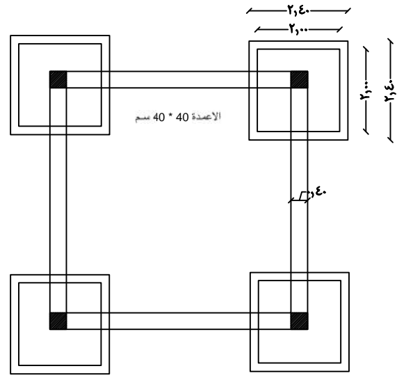
مسقط أفقى لارضية الخزان
