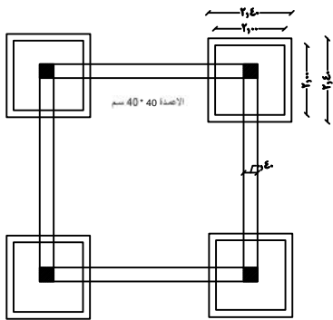
مسقط أفقي لارضية الخزان
