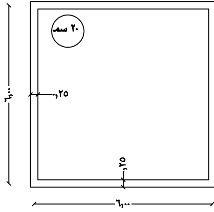
مسقط أفقى للسقف
