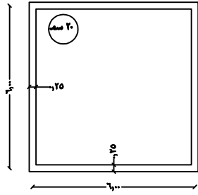
مسقط أفقي للسقف
